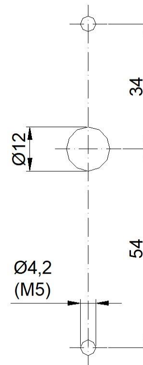
Bohrbild Maßstab 1:1
