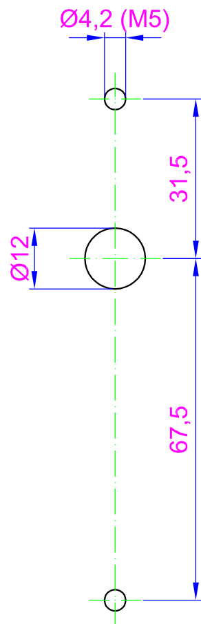
Bohrbild
