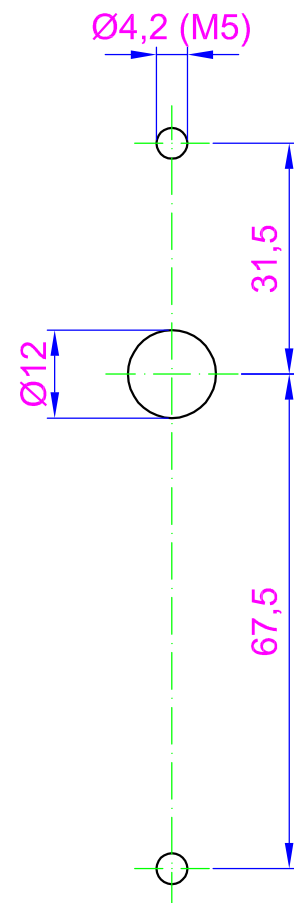
Bohrbild
